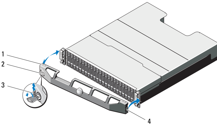
Abbildung 15-1. Frontverkleidung entfernen und anbringen
