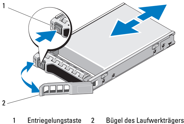
Abbildung 15-4. Laufwerk entfernen und installieren
