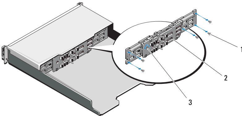
1 Schrauben (5) 2 Rückwandplatine 3 Selbstsichernde Schraube
