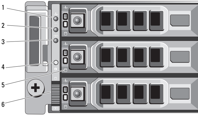
Abbildung 2-2. Funktionen und Anzeigen auf der Vorderseite – Dell PowerVault MD3200
