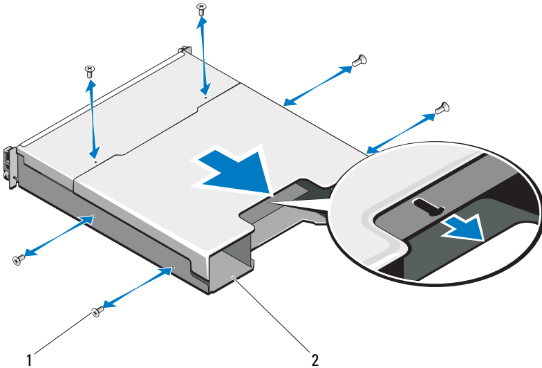
1 Schrauben (6) 2 RAID-Controller-Modul/Netzteilgehäuse
