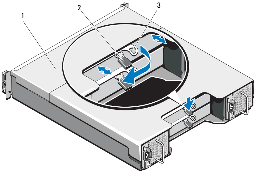
Abbildung 15-8. Entfernen und Installieren eines RAID-Controller-Moduls
