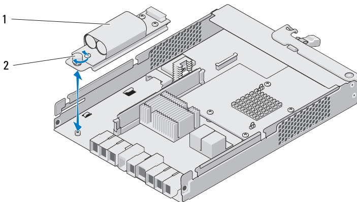
Abbildung 15-10. Entfernen und Installieren des RAID-Controller-Modul-Akkusicherungsmoduls
