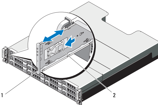
Abbildung 15-13. Entfernen und Installieren der Bedienfeldplatine – PowerVault MD3200
